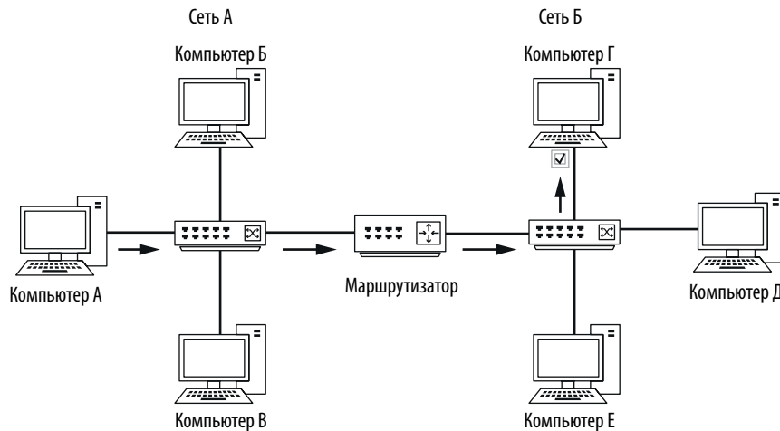
Рис. 1.10. Порядок прохождения сетевого трафика, когда компьютер А в одной сети передает данные компьютеру Г в другой сети через маршрутизатор
