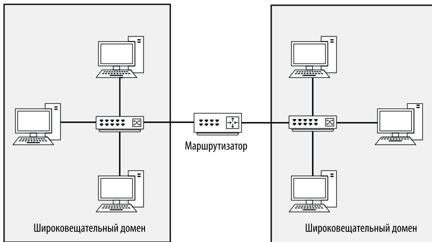
Рис. 1.11. Широковещательный домен охватывает весь текущий сегмент маршрутизируемой сети до маршрутизатора
