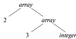
Рис. 5.15. Выражение типа для int [2] [3]
