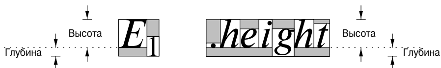
Рис. 5.24. Построение больших боксов из меньших
