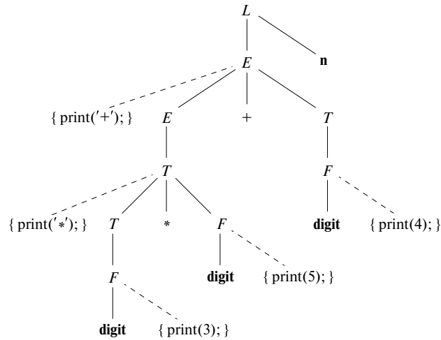
Рис. 5.22. Дерево разбора с добавленными действиями
